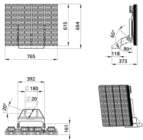
Габаритный чертеж
