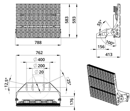
Габаритный чертеж
