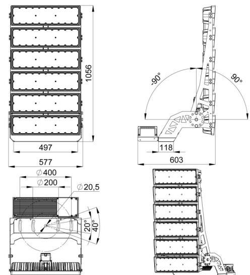
Габаритный чертеж
