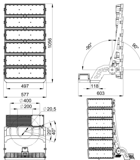
Габаритный чертеж
