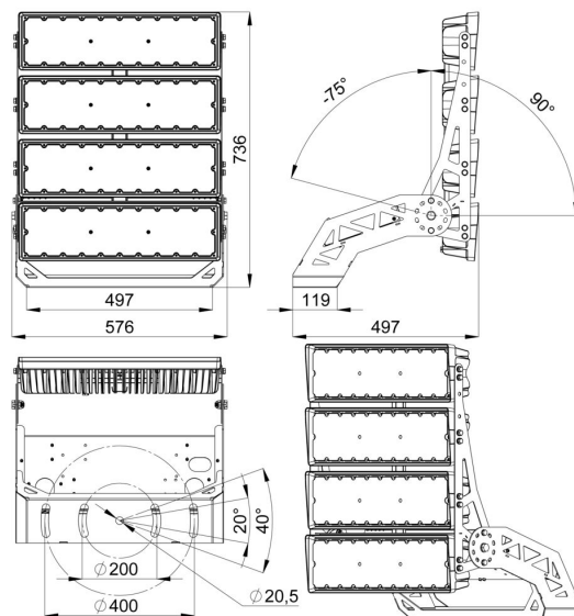
Габаритный чертеж
