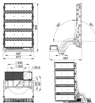
Габаритный чертеж
