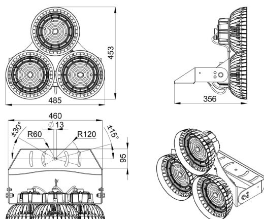
Габаритный чертеж
