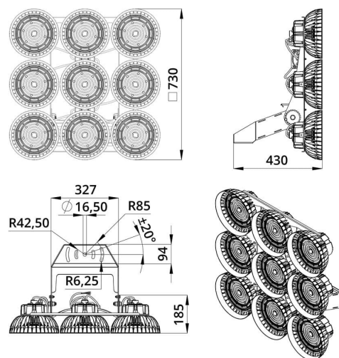
Габаритный чертеж
