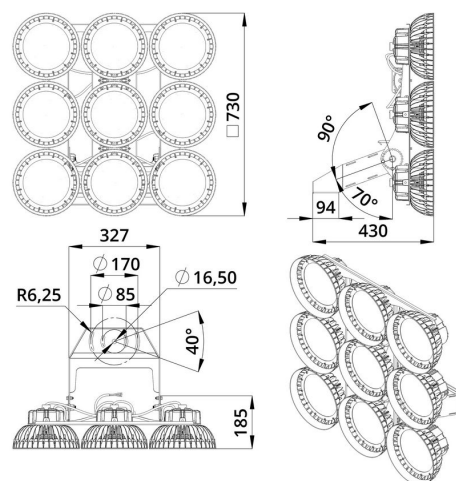
Габаритный чертеж
