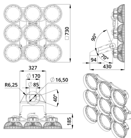
Габаритный чертеж
