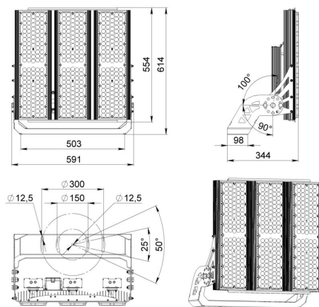
Габаритный чертеж
