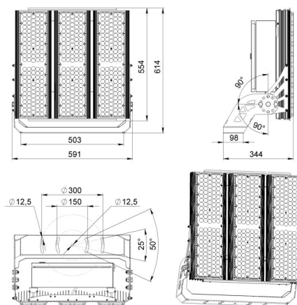
Габаритный чертеж
