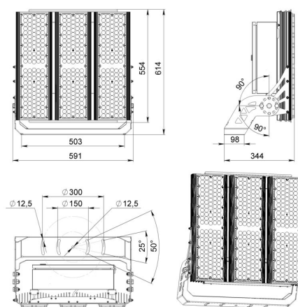
Габаритный чертеж
