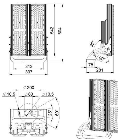
Габаритный чертеж
