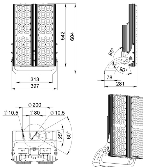
Габаритный чертеж
