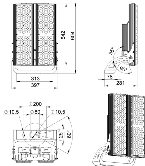
Габаритный чертеж
