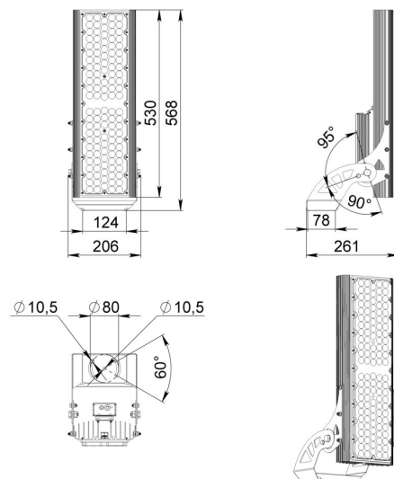
Габаритный чертеж
