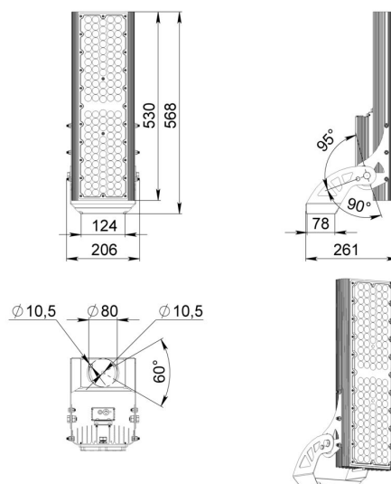
Габаритный чертеж
