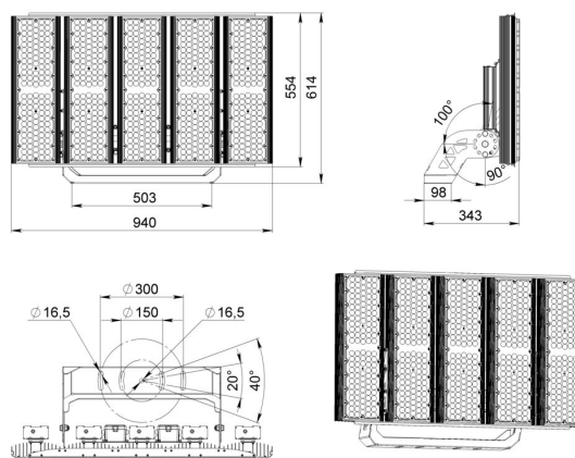
Габаритный чертеж
