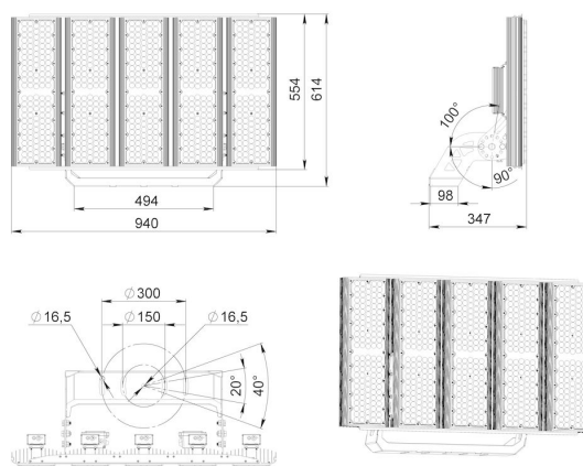
Габаритный чертеж
