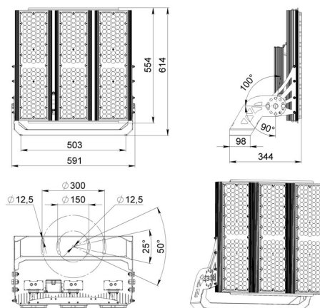
Габаритный чертеж
