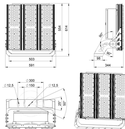
Габаритный чертеж
