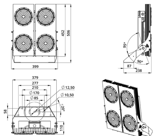
Габаритный чертеж
