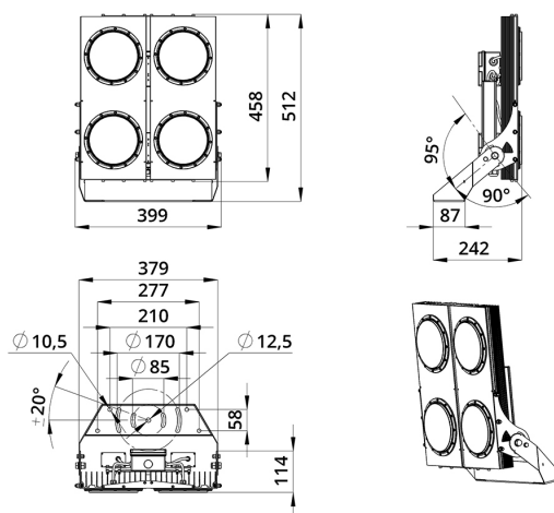
Габаритный чертеж
