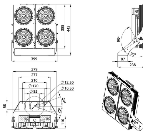
Габаритный чертеж
