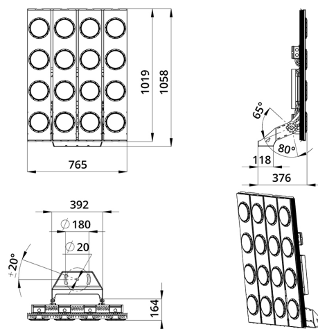
Габаритный чертеж
