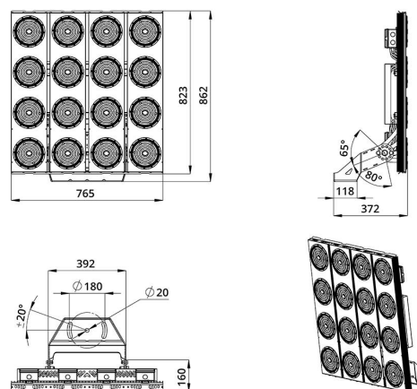
Габаритный чертеж
