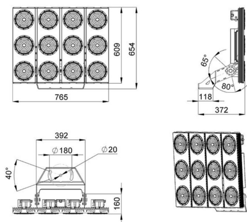
Габаритный чертеж
