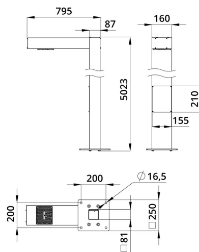
Габаритный чертеж
