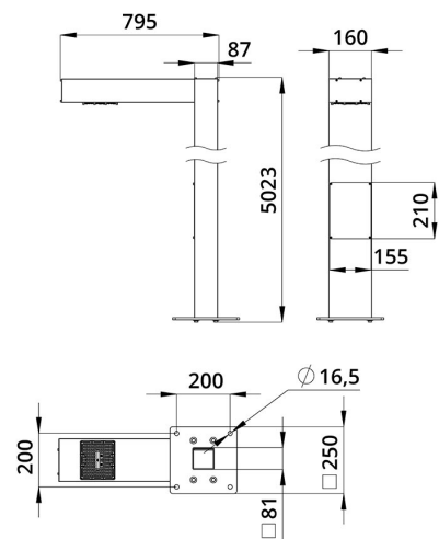
Габаритный чертеж
