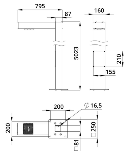
Габаритный чертеж
