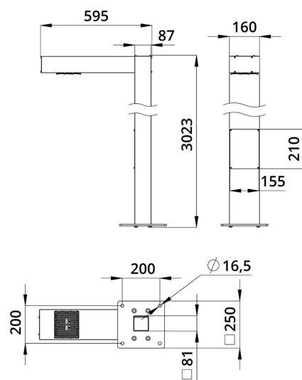
Габаритный чертеж
