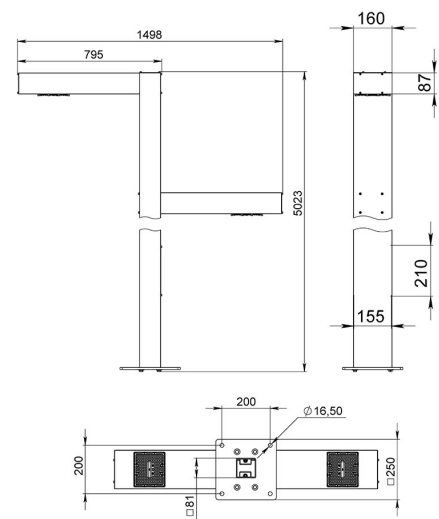
Габаритный чертеж
