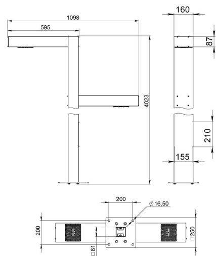
Габаритный чертеж
