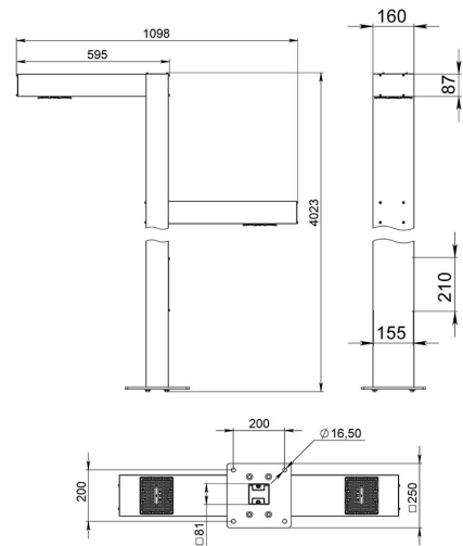
Габаритный чертеж
