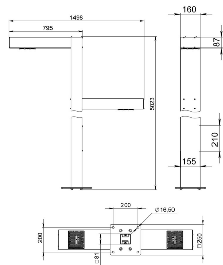
Габаритный чертеж
