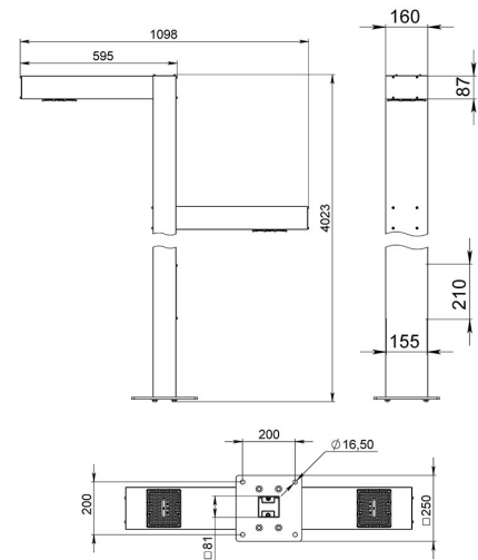
Габаритный чертеж
