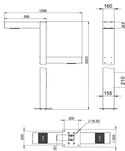
Габаритный чертеж
