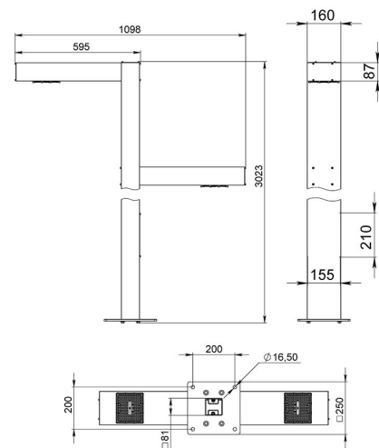
Габаритный чертеж
