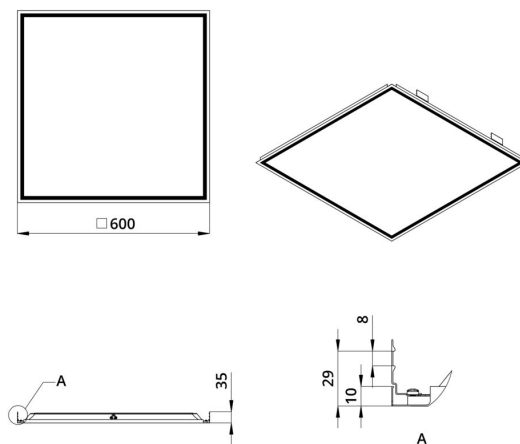
Габаритный чертеж
