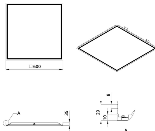
Габаритный чертеж
