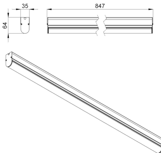
Габаритный чертеж
