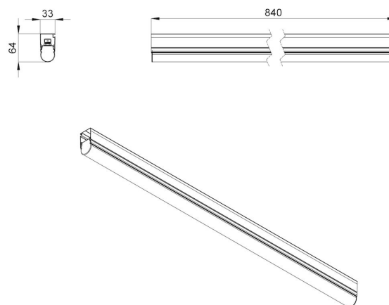
Габаритный чертеж
