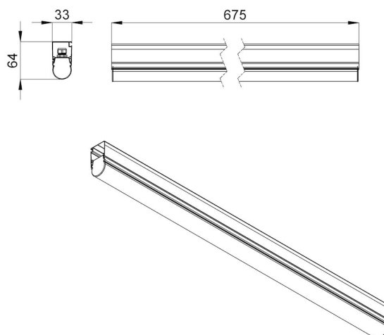
Габаритный чертеж
