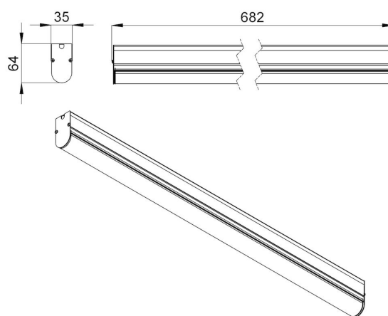
Габаритный чертеж
