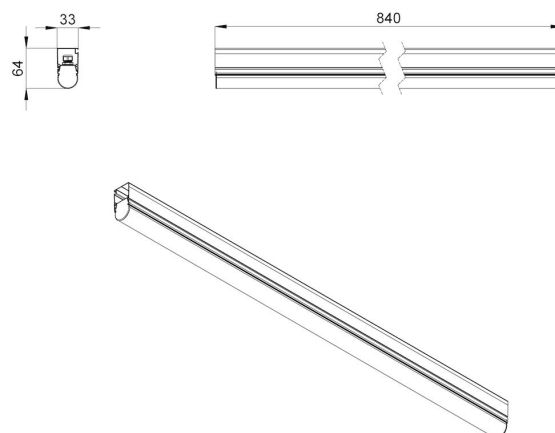
Габаритный чертеж
