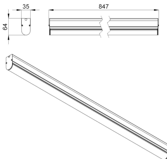
Габаритный чертеж
