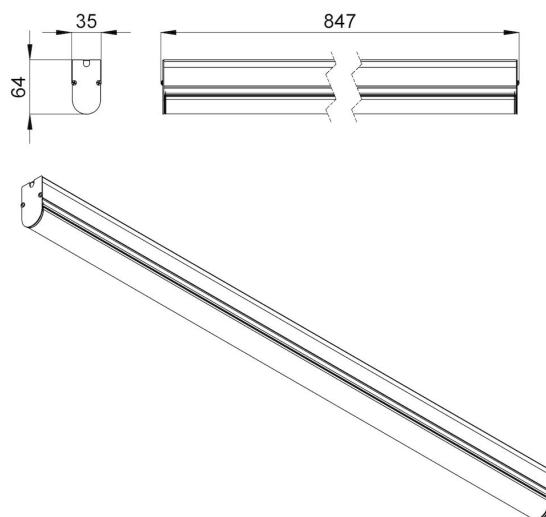
Габаритный чертеж
