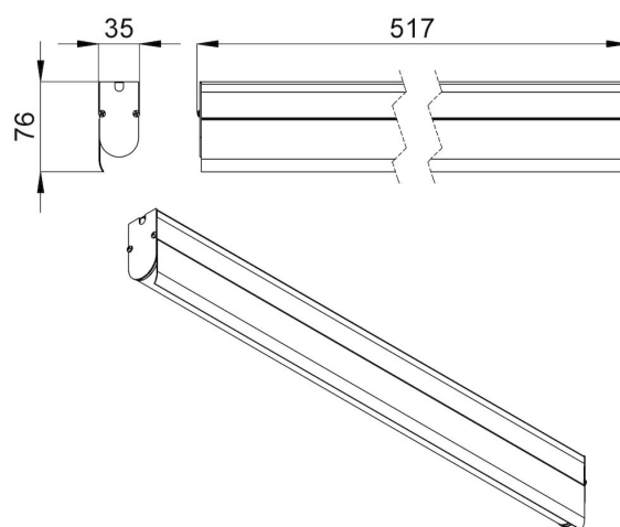
Габаритный чертеж
