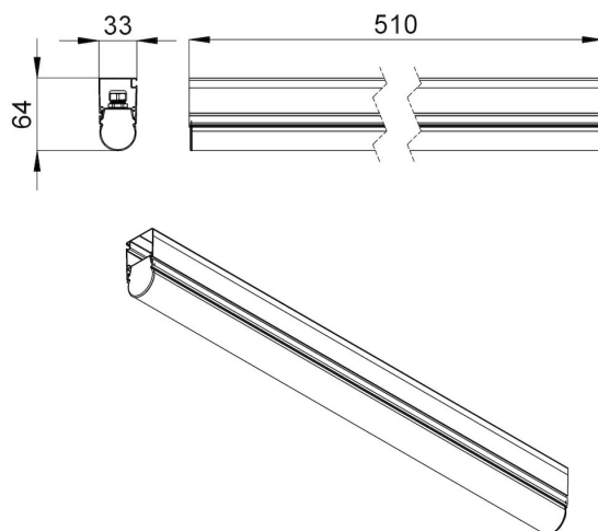
Габаритный чертеж
